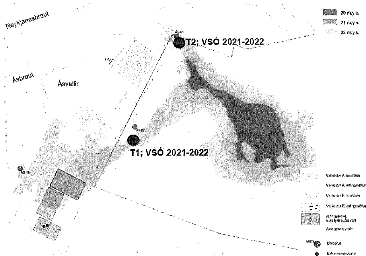
Mynd 8.2. Hæðarlínugreining af Ástjörn. Við hækkun vatnsyfirborðs í Ástjörn beintist útrænslið til vesturs og getur vatnsborð Ástjarnar því ekki orðið hærra en ca. 21 m y.s.
